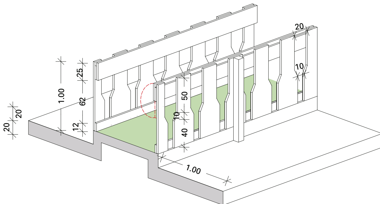
AXONOMETRIE
